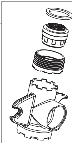
RP102039 Aerator & Wrench Aireador y Llave Aérateur et Clé
