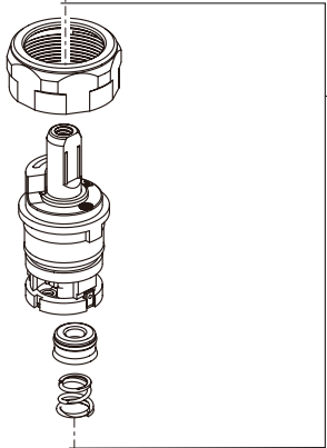
RP101504 Stem Unit Assembly, Seat & Spring, Bonnet Nut Ensamble de la Unidad del Vástago, Asiento y Resorte, Bonete Obturbateur, siège et ressort, écrou à chapeau
